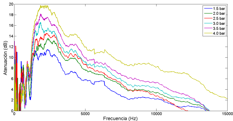
Figura 2. Atenuación sonora de los difusores simples de tipo TP11004 a distintas presiones.
