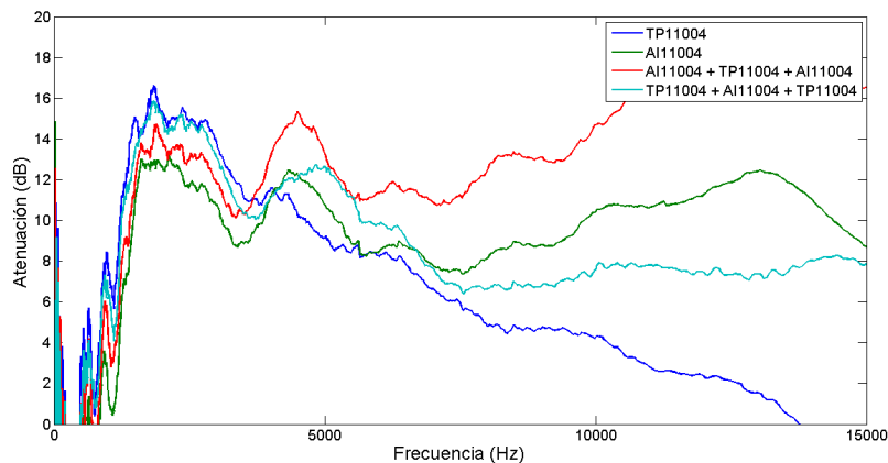
Figura 15. Comparación de la atenuación sonora de distintas combinaciones de difusores a la presión de 3,0 bar.
